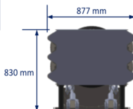
SIDE ELEVATION (TL2 & TL3)
